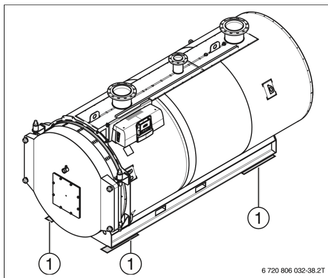
Рисунок 12 Укладка звукоизоляционных полос
