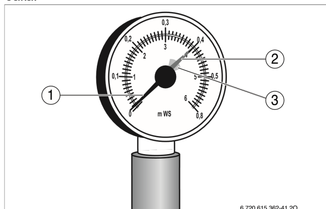
Рисунок 28 Манометр для открытых отопительных установок
