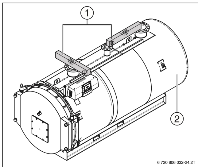
Рисунок 11 Выравнивание котла
