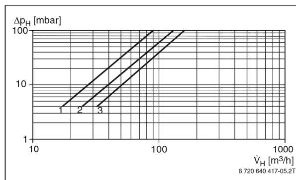
Рисунок 6 Гидравлическое сопротивление котлов SK 730 - 1850 кВт
