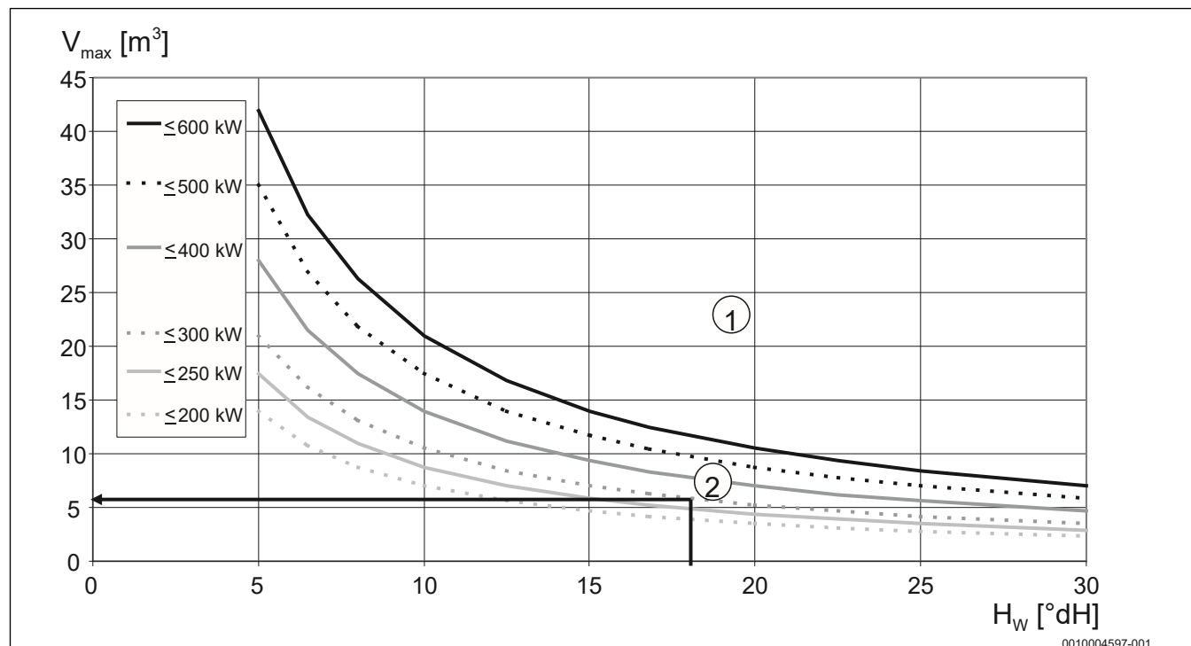
Рисунок 32 Требования к воде для заполнения и подпитки котлов из черных металлов мощностью от 200 до 600 кВт
