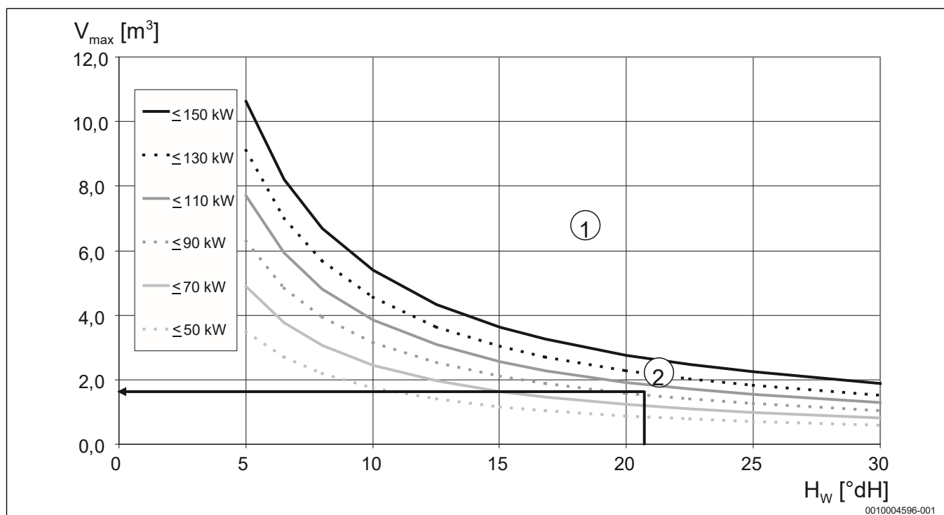
Рисунок 31 Требования к воде для заполнения и подпитки котлов из черных металлов мощностью до 150 кВт
