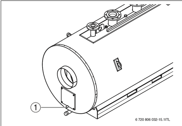
Рисунок 27 Закрытие/открытие стока для чистящих средств
