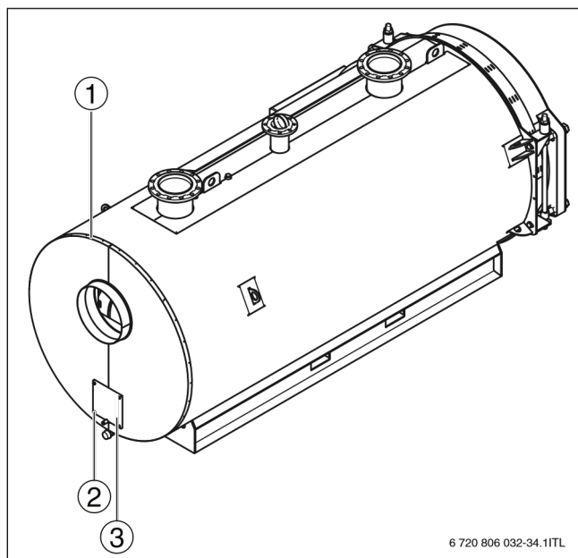
Рисунок 26 Установка крышки люка для чистки
