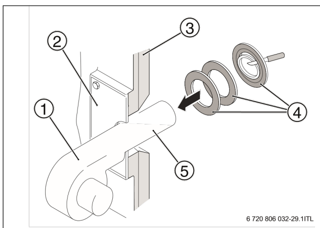
Рисунок 18 Монтаж горелки
