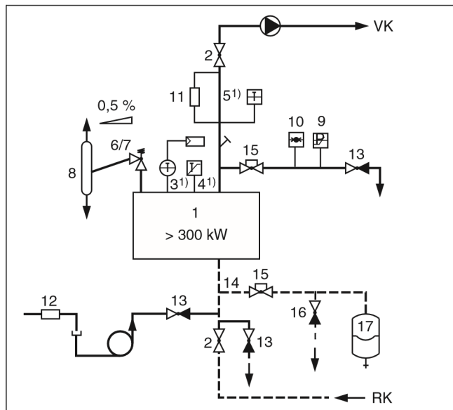
Рисунок 30 Приборы безопасности для котла для котла > 300 кВт с STB \leq 110^\circ\text{C} (прямой нагрев)
