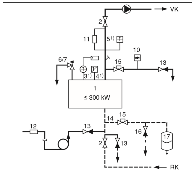
Рисунок 29 Приборы безопасности для котла для котла \leq 300 кВт с STB \leq 110^\circ\text{C} (прямой нагрев)
