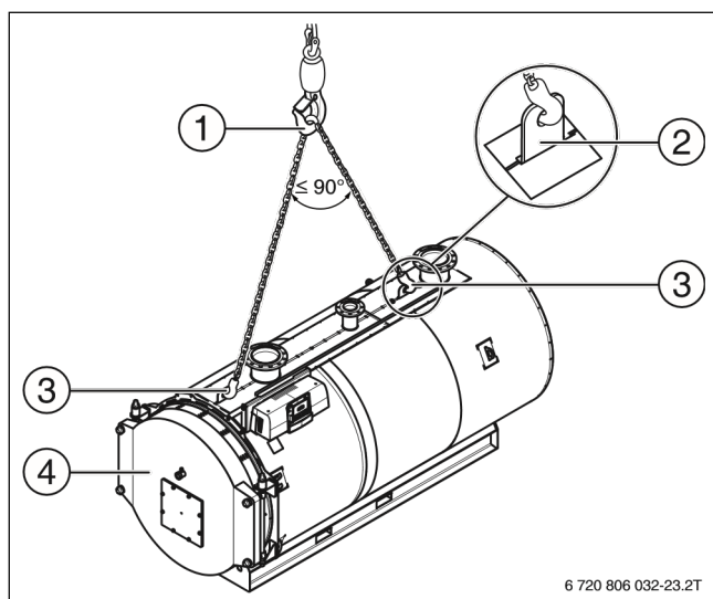
Рисунок 9 Схема строповки
